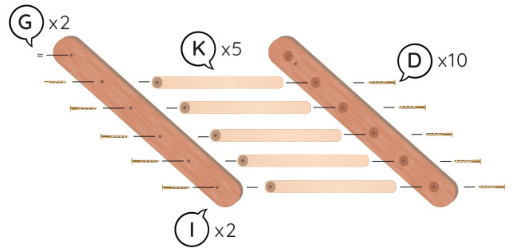
VUE PETIT CÔTÉ ASSEMBLÉ
